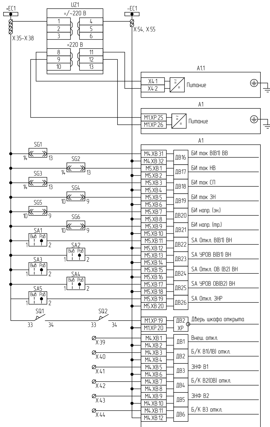
Питание оперативных цепей Питание ИЧМ Питание ИЗУ Контроль положения испытательных блоков Контроль положения переключателей Контроль положения дверей шкафа Внешнее отключение Положение В1 ЗНФ В1 Положение В2 ЗНФ В2 Положение В3
