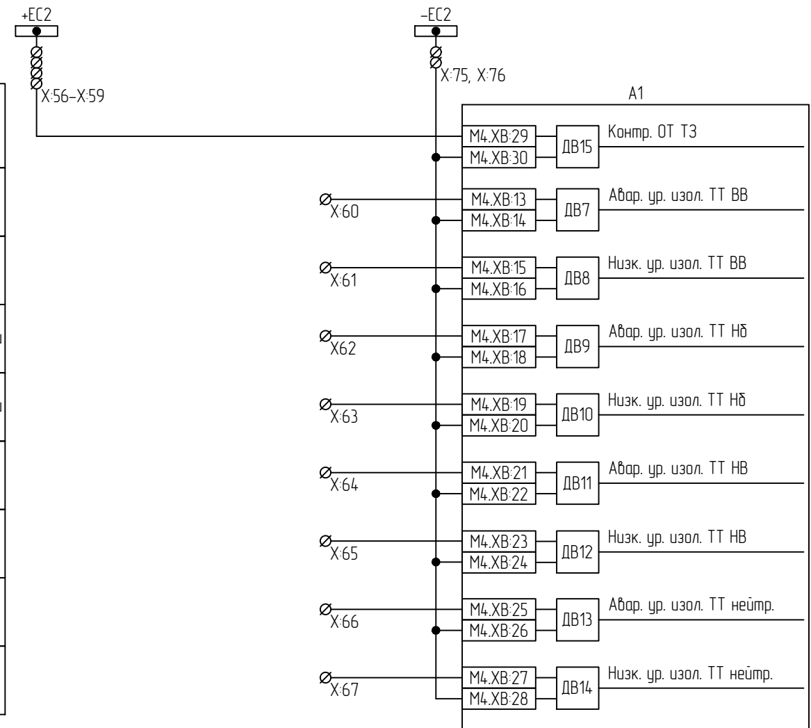
Контроль оперттока технологической сигнализацции Аварийный уровень изоляции ТТ ВН БСК Низкий уровень изоляции ТТ ВН БСК Аварийный уровень изоляции ТТ средней перемычки Низкий уровень изоляции ТТ средней перемычки Аварийный уровень изоляции фазных ТТ нейтрал Низкий уровень изоляции фазных ТТ нейтрал Аварийный уровень изоляции ТТ нейтрал Низкий уровень изоляции ТТ нейтрал
